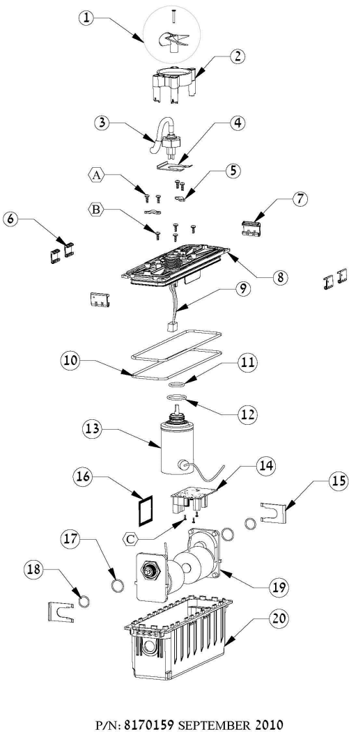
#12 MOTOR UNIT CATALOG KIT C3/C4
